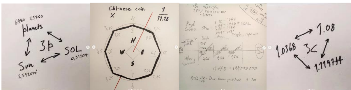
Constantes clés CHI W-n-e-se E/M=C2 Constantes clés
