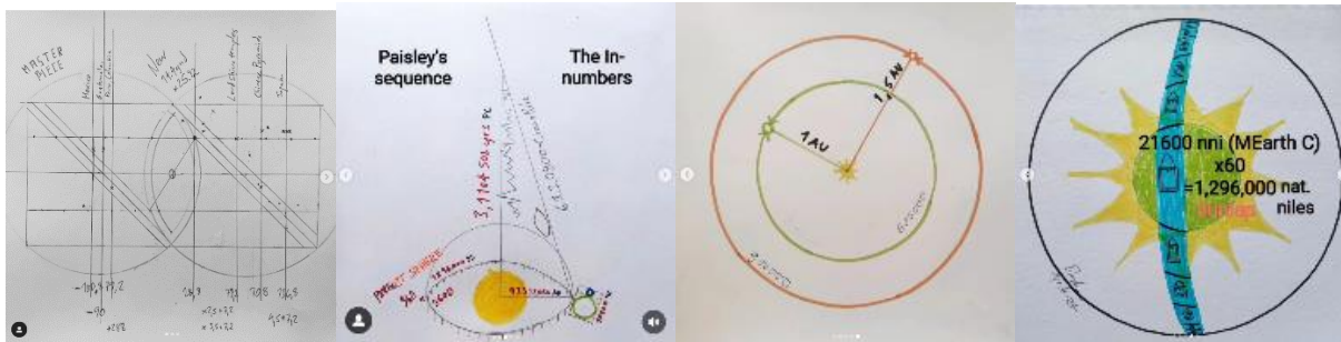
Latitude 288° 3.1104 (Parsec) M Earth, Mars AU ratio Soleil Soleil lap 1,296,000 nn
